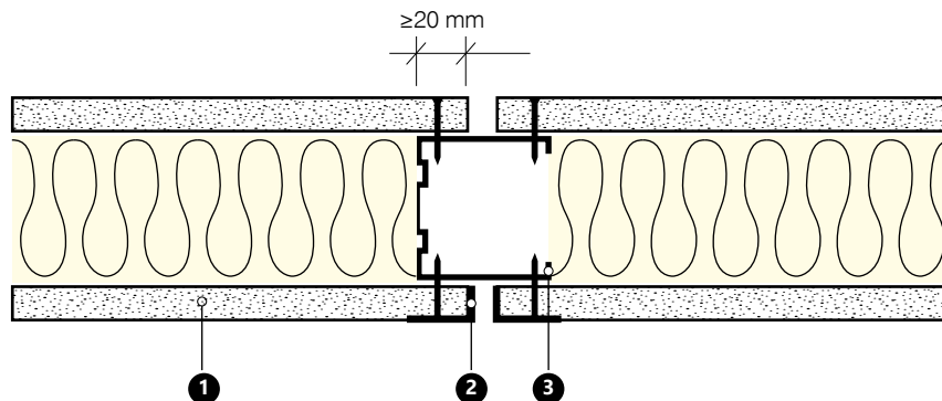
Fig. 42. Open gap.
